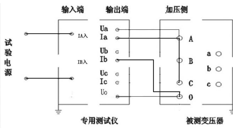
图二十九 零序阻抗接线图
