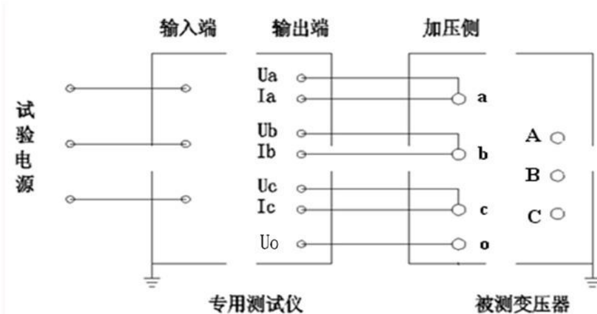
图二十 变压器三相空载测试接线图
