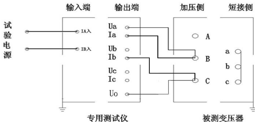
图二十四 单相负载接线图
