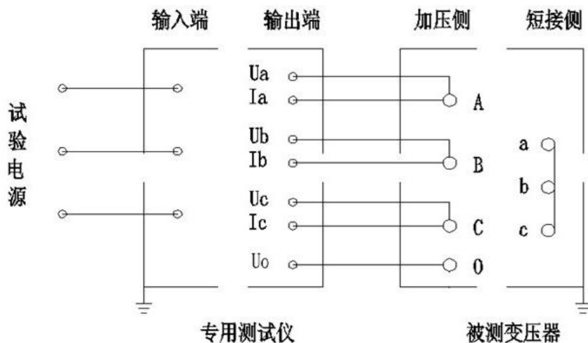
图十七 变压器三相负载测试接线图
